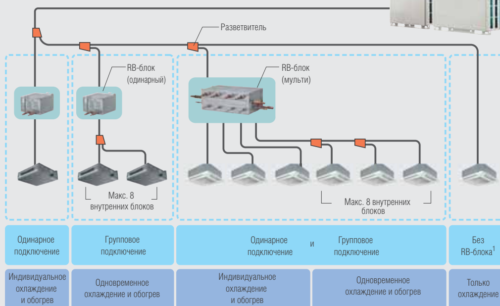
RB-блок (одинарный)
